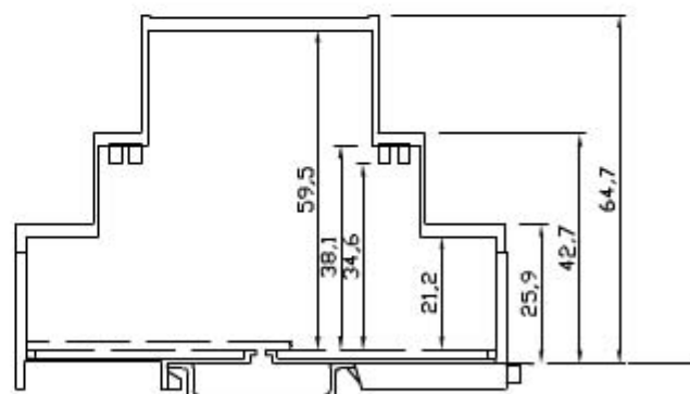
BARRA DIN
