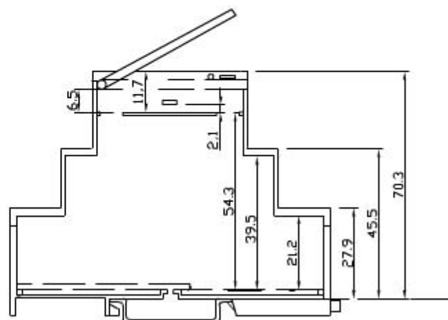
BARRA DIN
