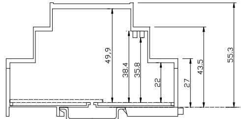
BARRA DIN
