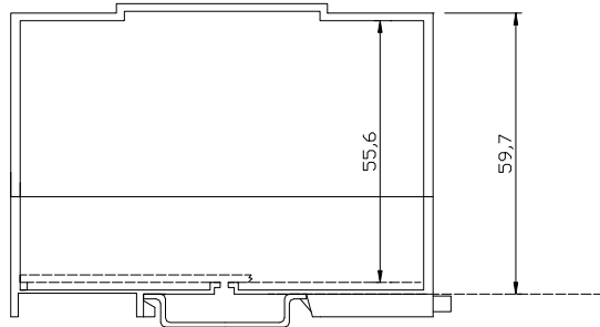
BARRA DIN
