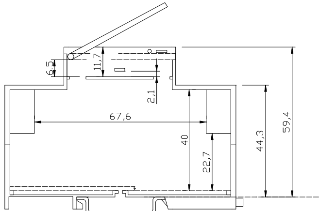
BARRA DIN
