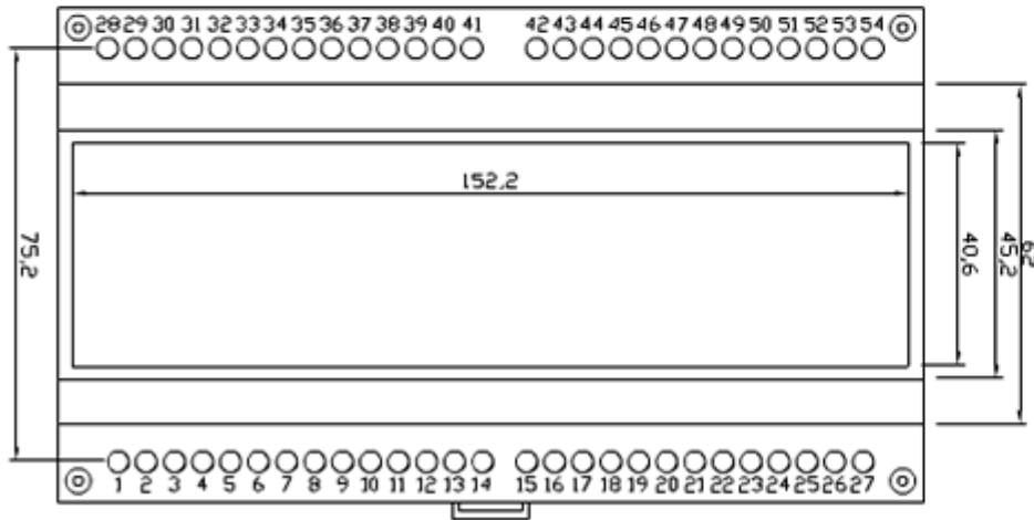
BARRA DIN
